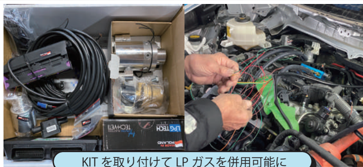
KIT を取り付けて LP ガスを併用可能に
